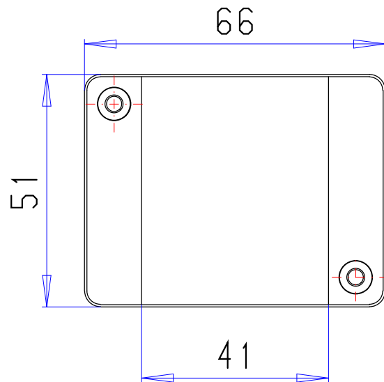
Ansicht mit Deckel
